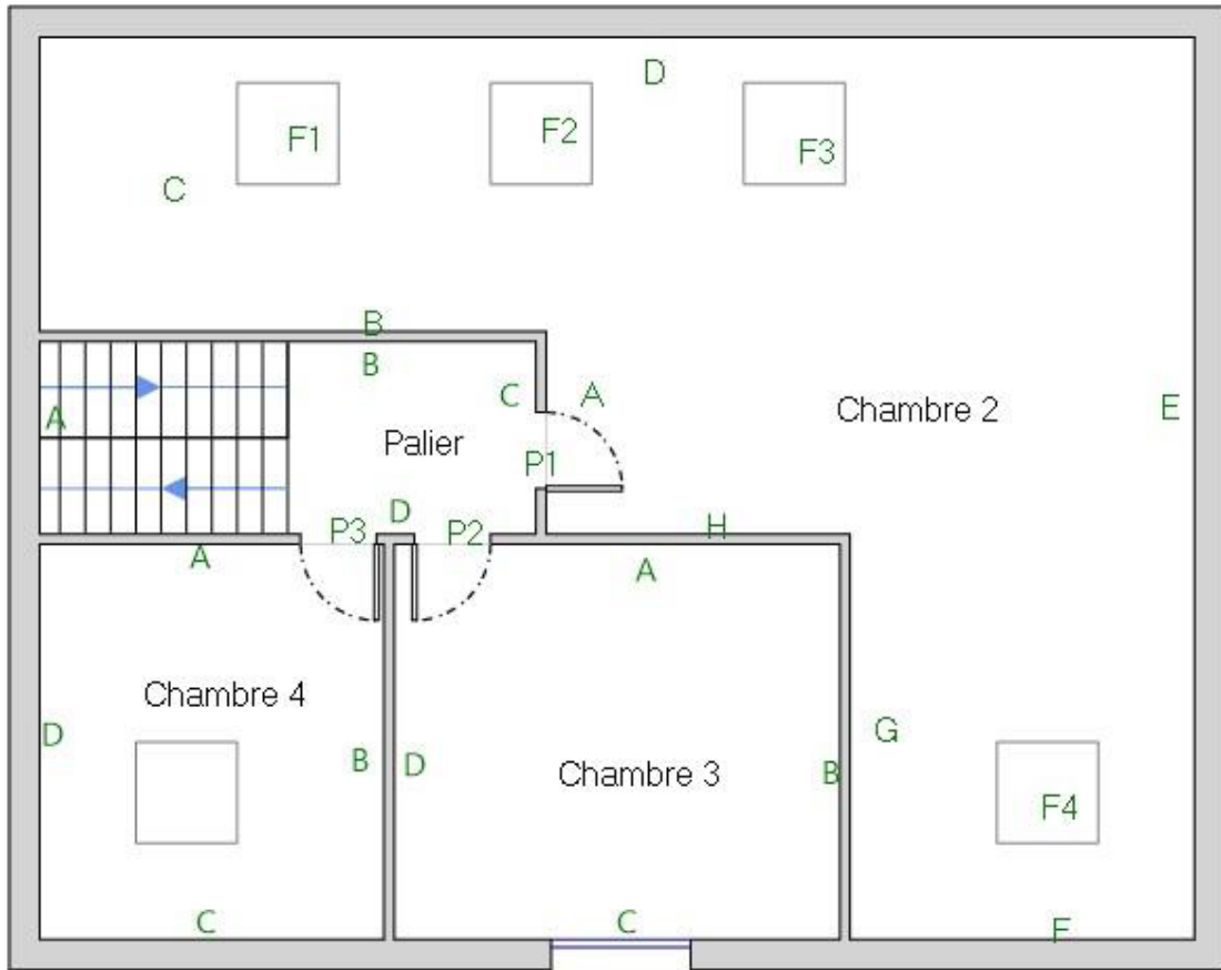
2ème Etage
